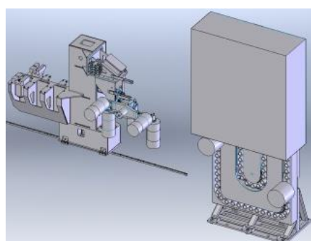
Magazzino ISO50/Capto con navetta porta pinze e teste
