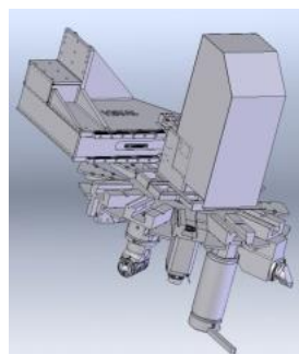
Magazzino 12 torrette
